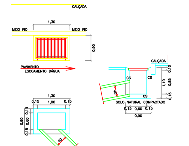
PLANTA BAIXA ESC. 1/75
