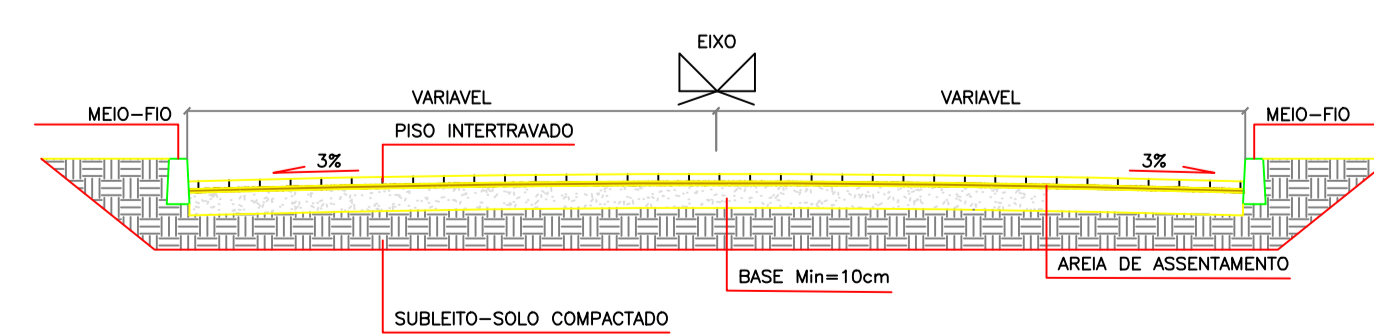
PERFIL DETALHE DE PAVIMENTAÇÃO PAVIES SOBRE TERRENO NATURAL – ESC. 1/50
