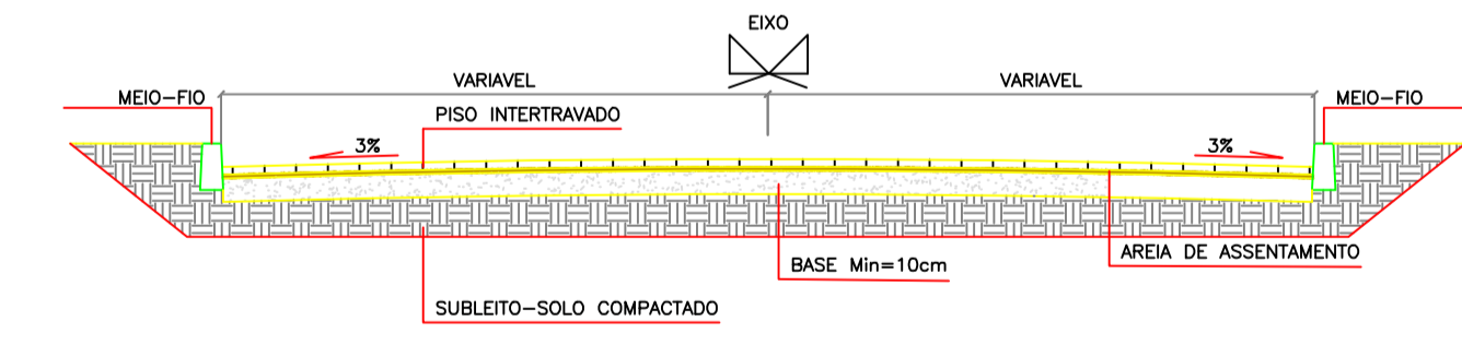
PERFIL DETALHE DE PAVIMENTAÇÃO PAVIES SOBRE TERRENO NATURAL - ESC. 1/50
