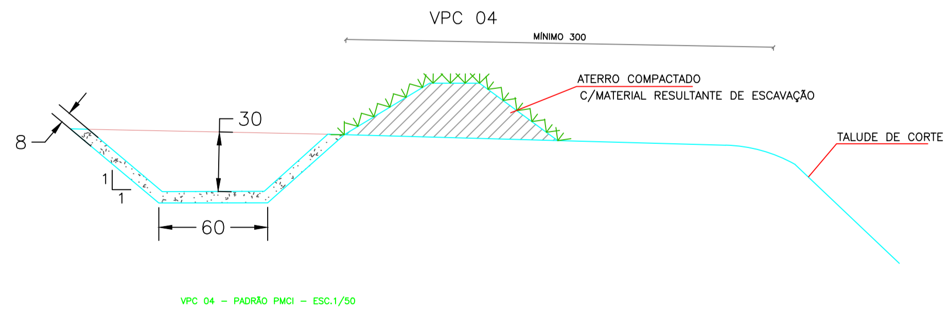
VPC 04 - PADRÃO PMCI - ESC. 1/50
