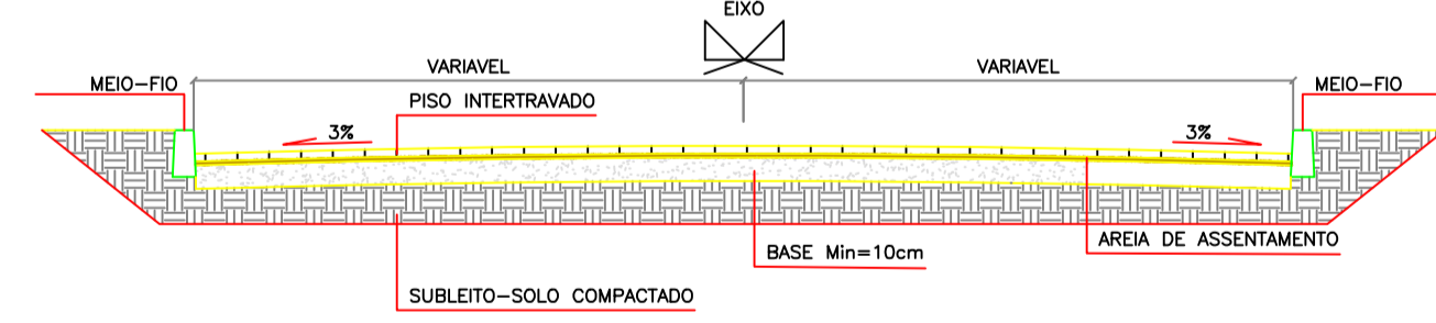
PERFIL DETALHE DE PAVIMENTAÇÃO PAVIES SOBRE TERRENO NATURAL - ESC. 1/50
