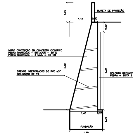
SEÇÃO B - MURO ESC.1/100
