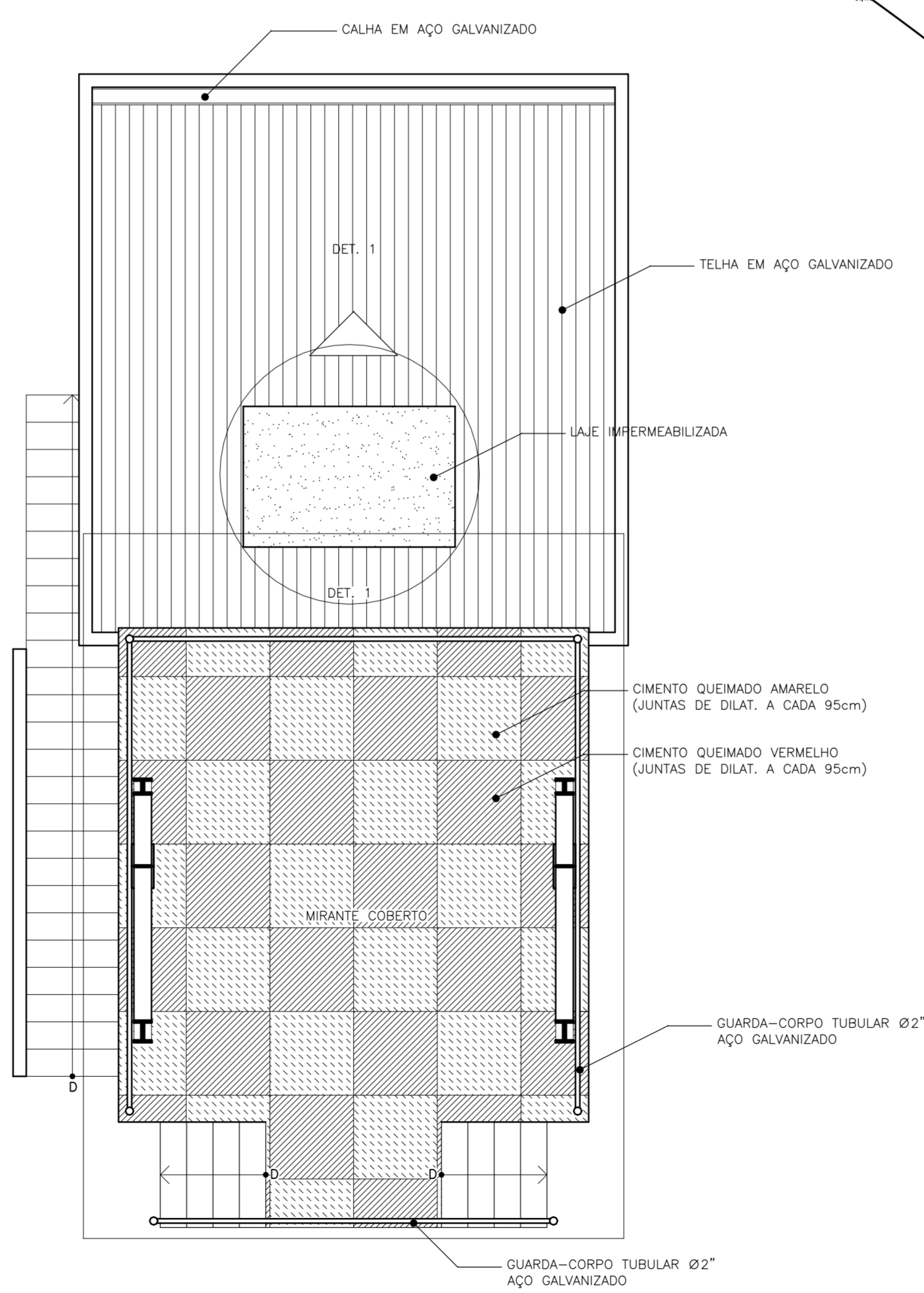
PLANTA COBERTURA – ESC. 1/50
